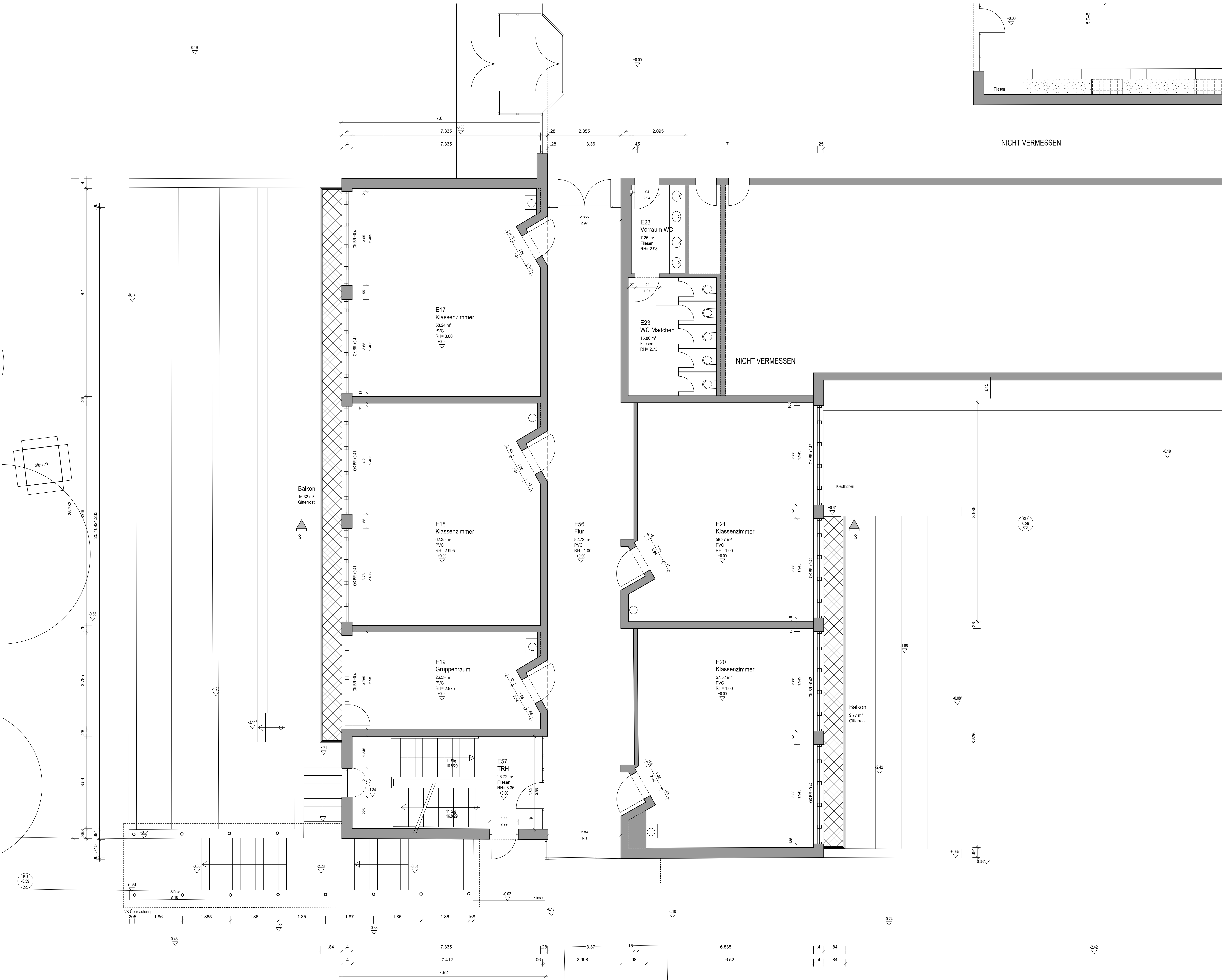
Grundriss EG
